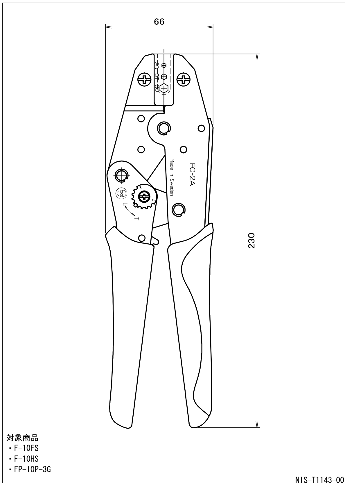
外観図 FC-2A
